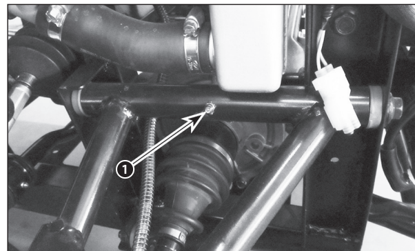
1. Пресс-масленка
