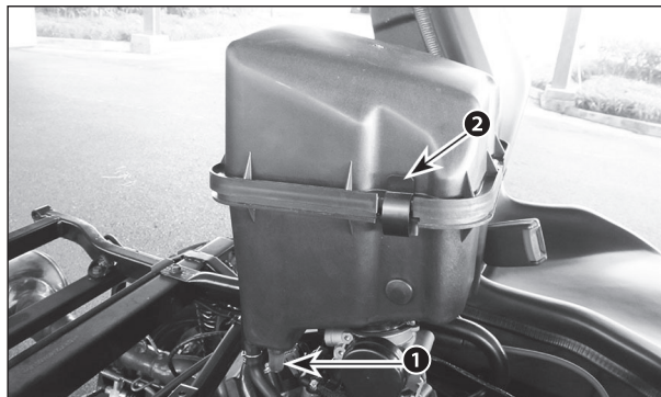
1. Трубка-отстойник
