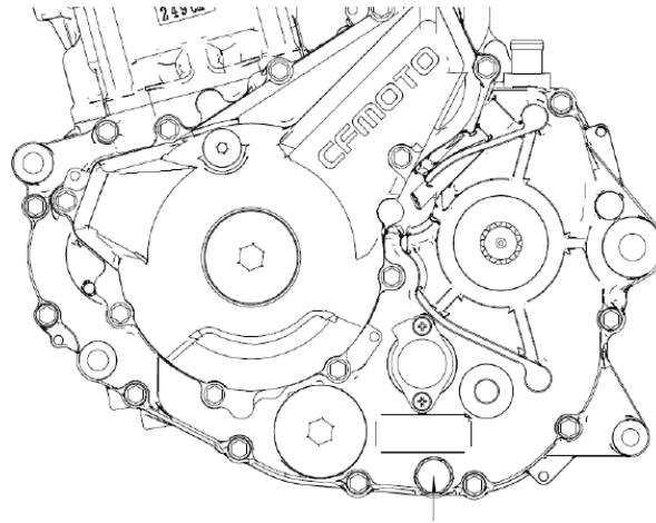
Сливная пробка
