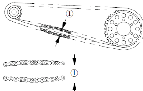
1. Провисание цепи
