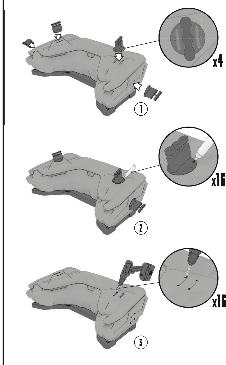
Установка канистр
