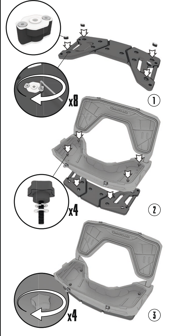
Установка кофра
