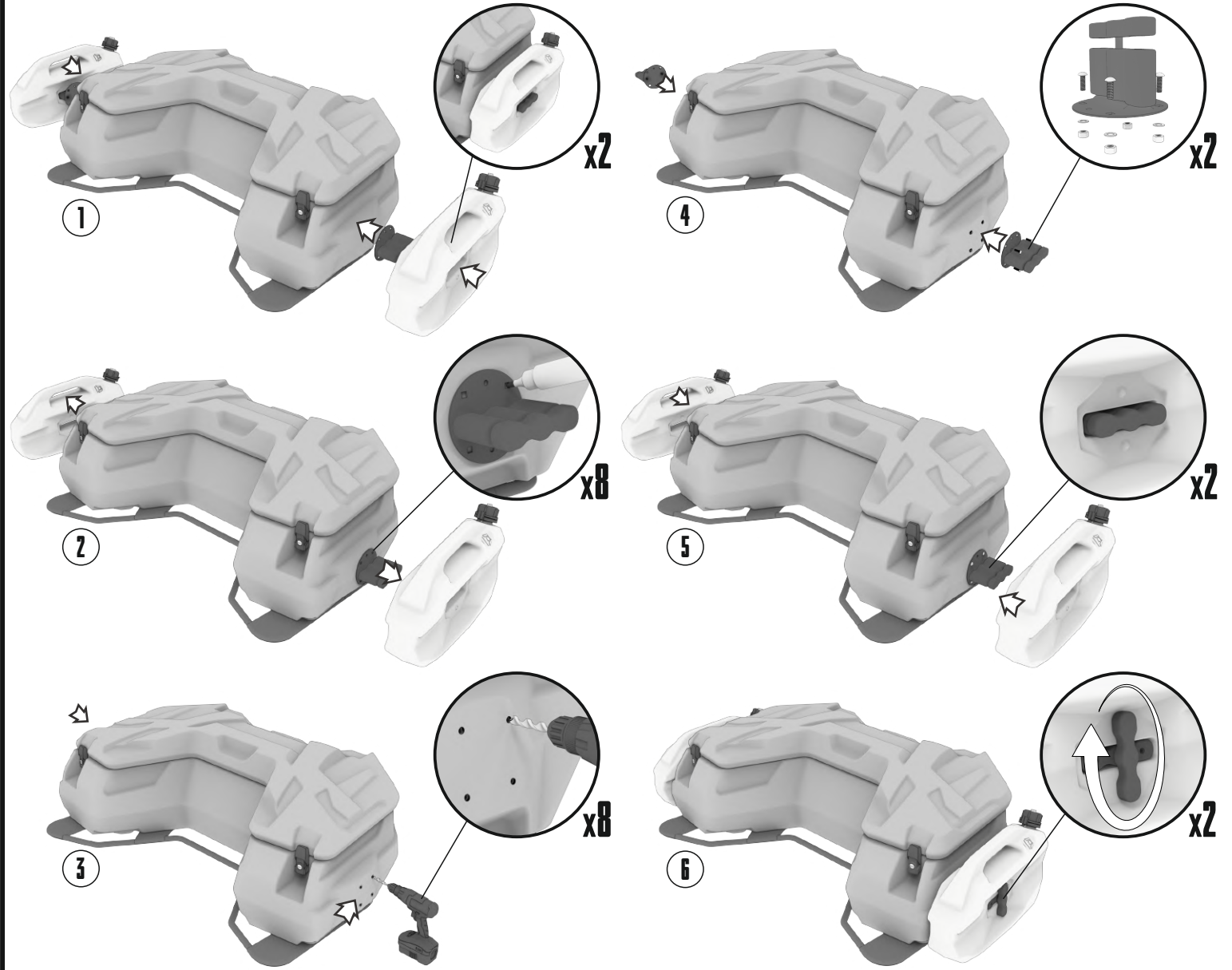
Установка канистр
