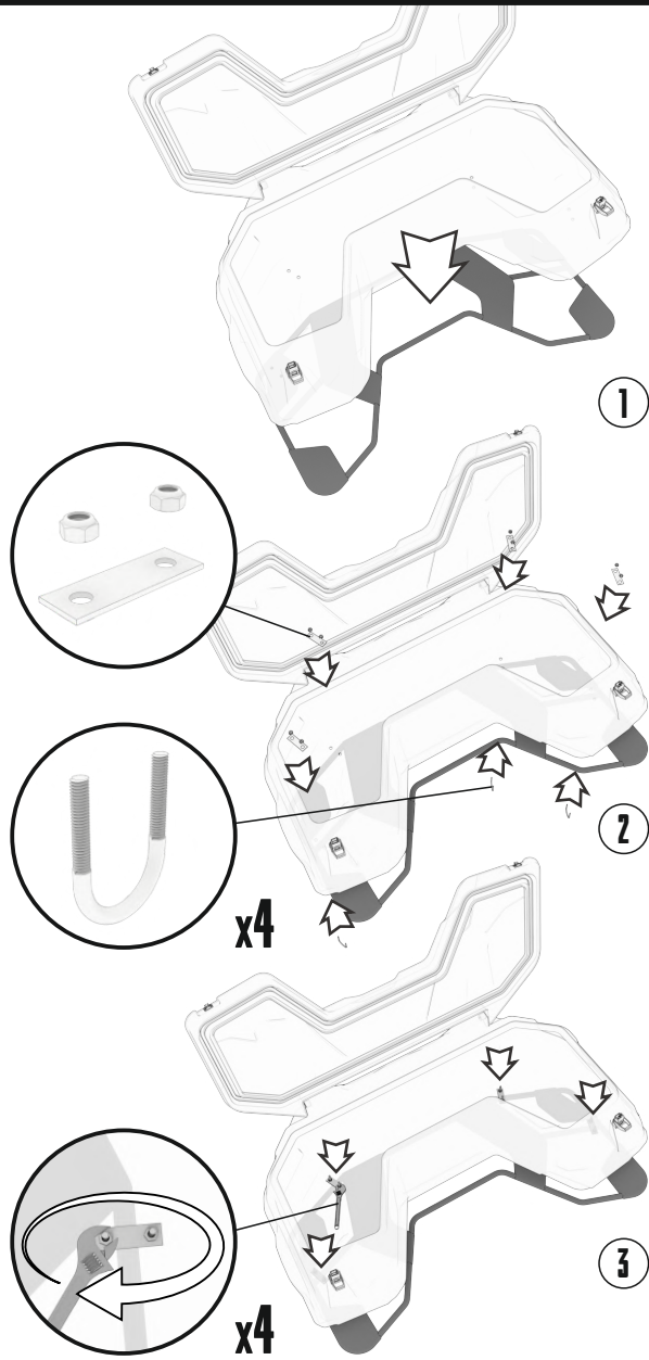
Установка кофра
