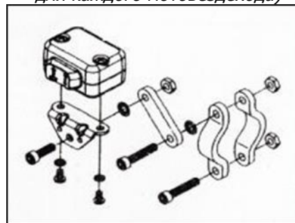
Установочный комплект переключателя направления вращения барабана лебедки
